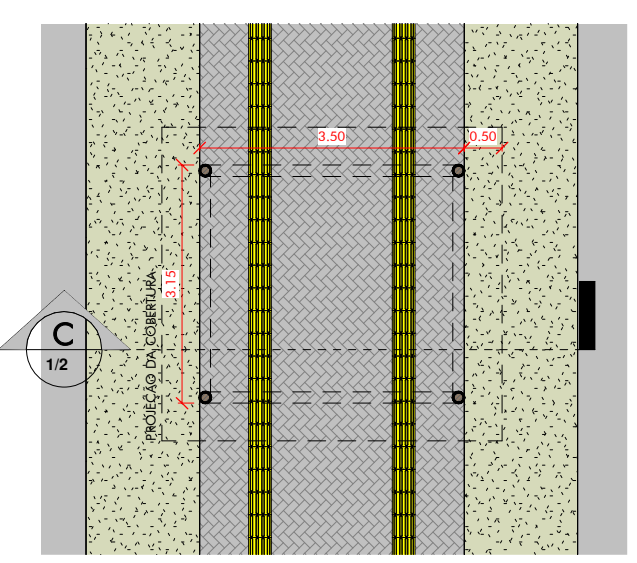
DETALHE DO QUIOSQUE
