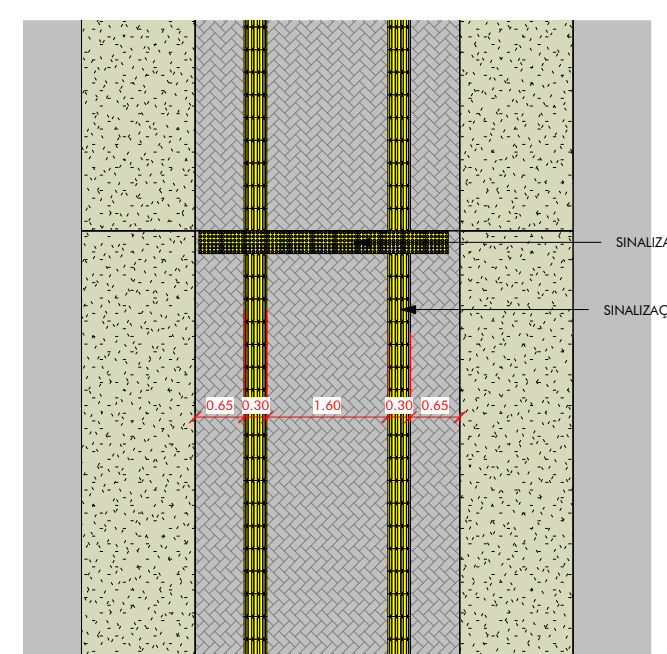
DETALHE PISO TÁTIL
