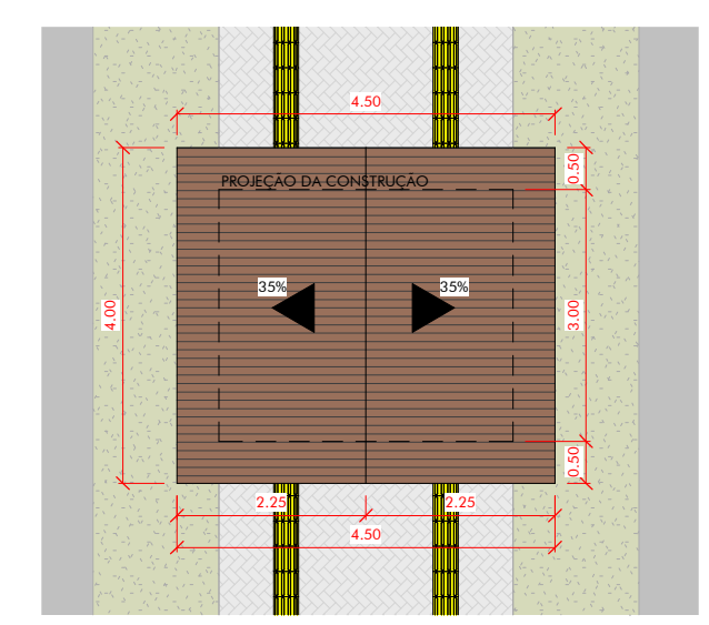
PLANTA COBERTURA
