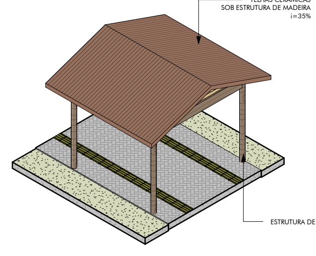
ISOMÉTRICO QUIOSQUE
