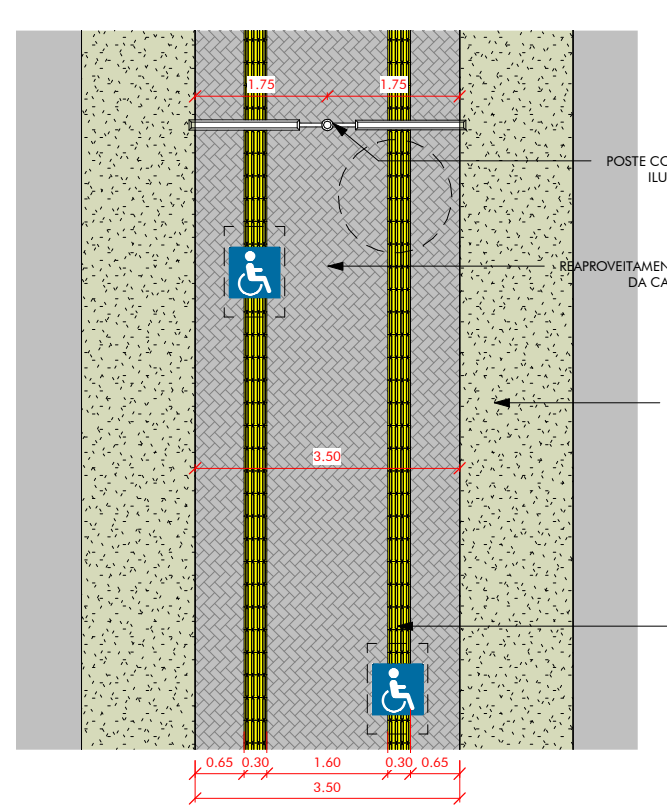
DETALHE DO PASSEIO
