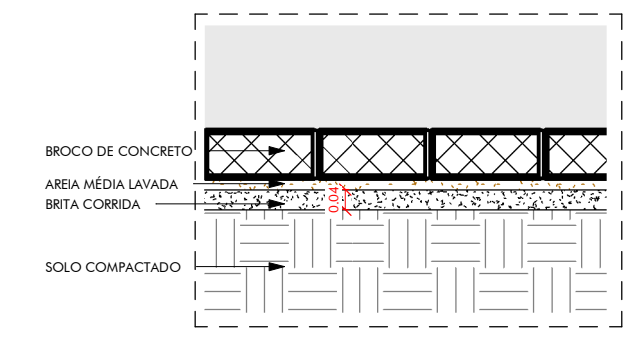
DETALHE DA CALÇADA
