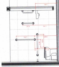
ELEVÇÃO B 1:50
