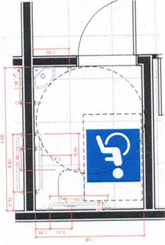
DETALHE WC PNE 1:10
